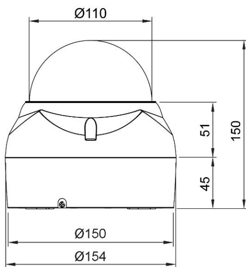
Вид спереди
