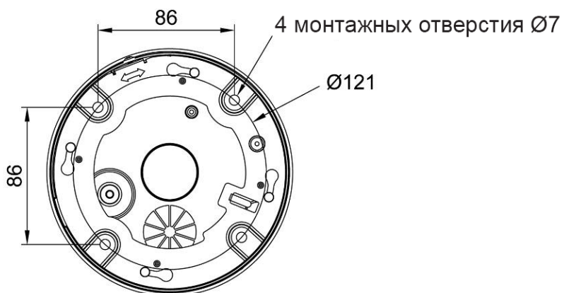
Вид снизу
